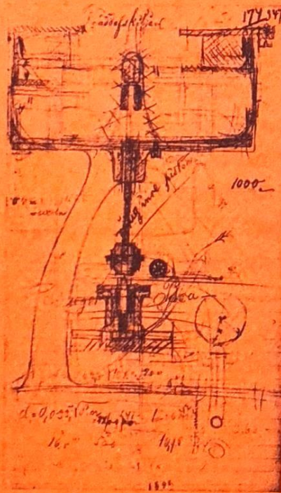
DEN FÖRSTA SKISSEN TILL DE LAVALS "GRÄDDAFSKILJARE" 1877
